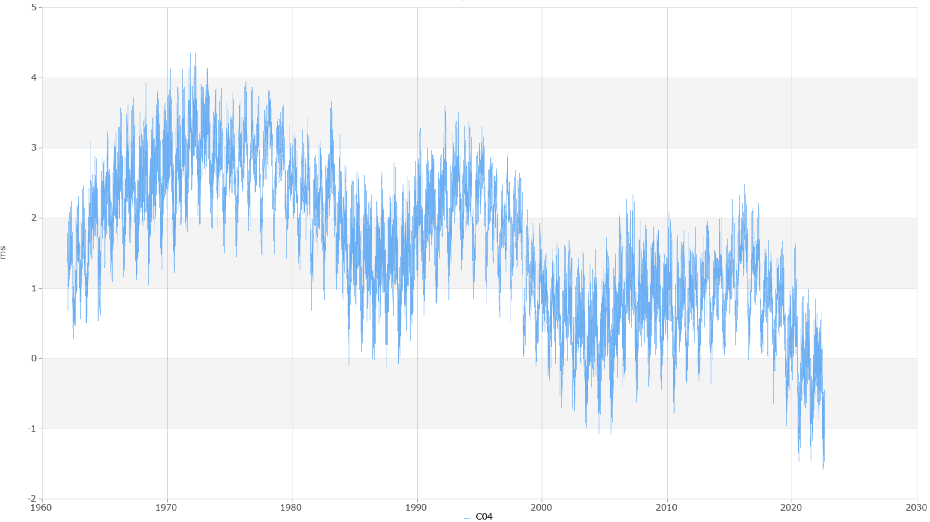
LOD / 86400 s SI
