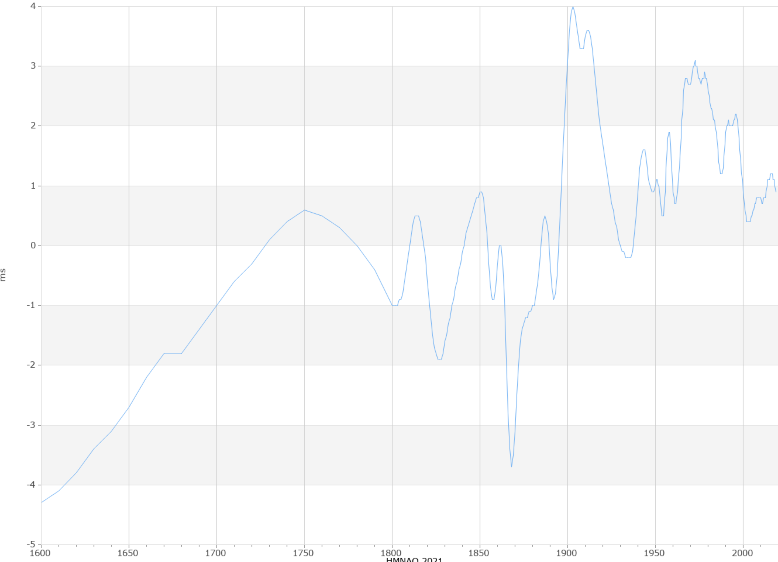
LOD / 86400 s SI
