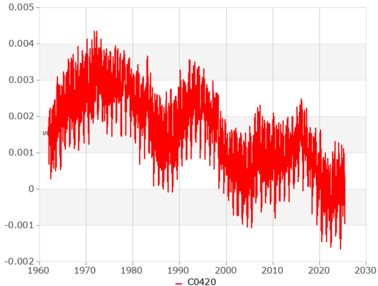
LOD / 86400 s SI
