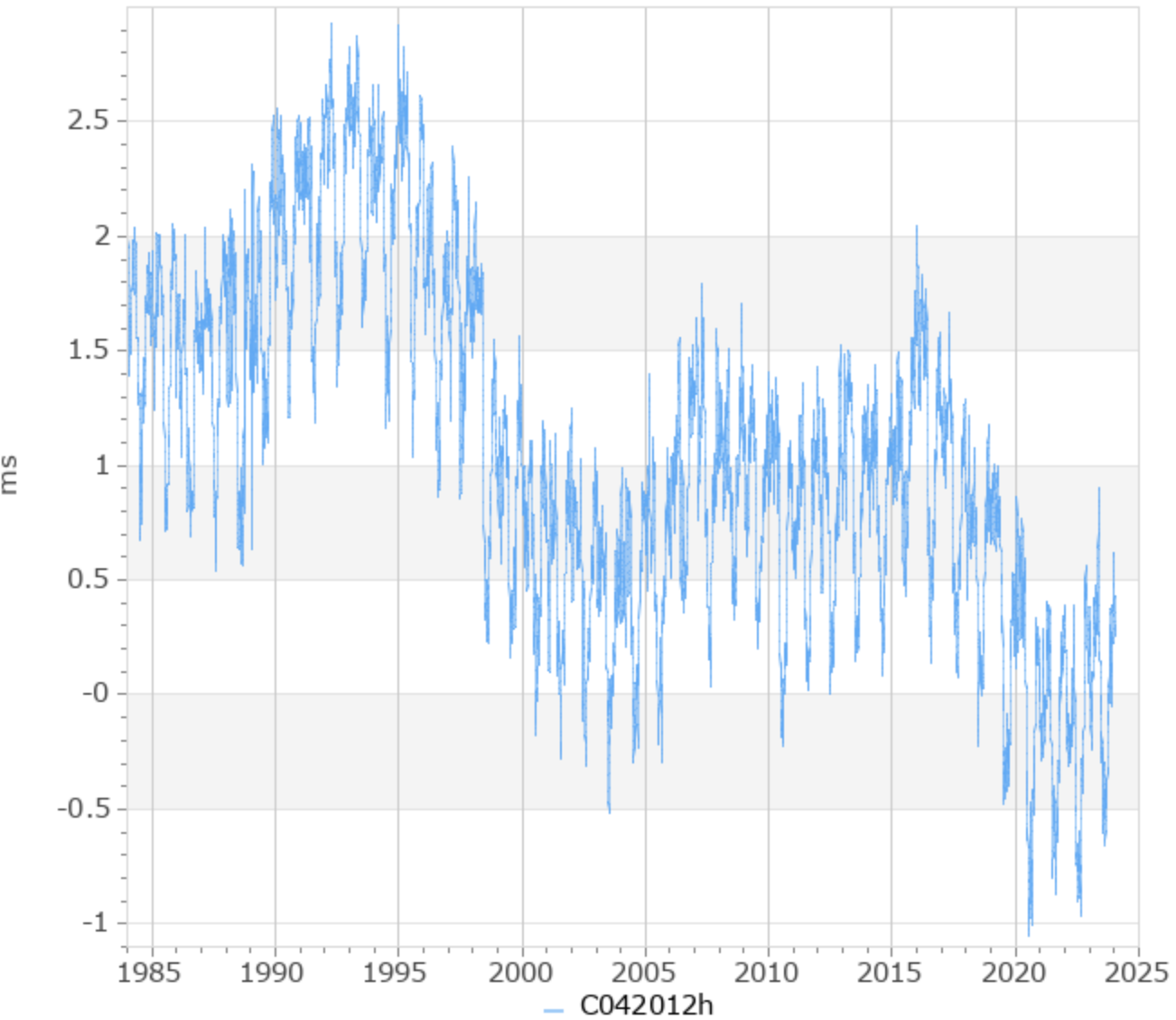
Durée du jour / 86400 s SI
