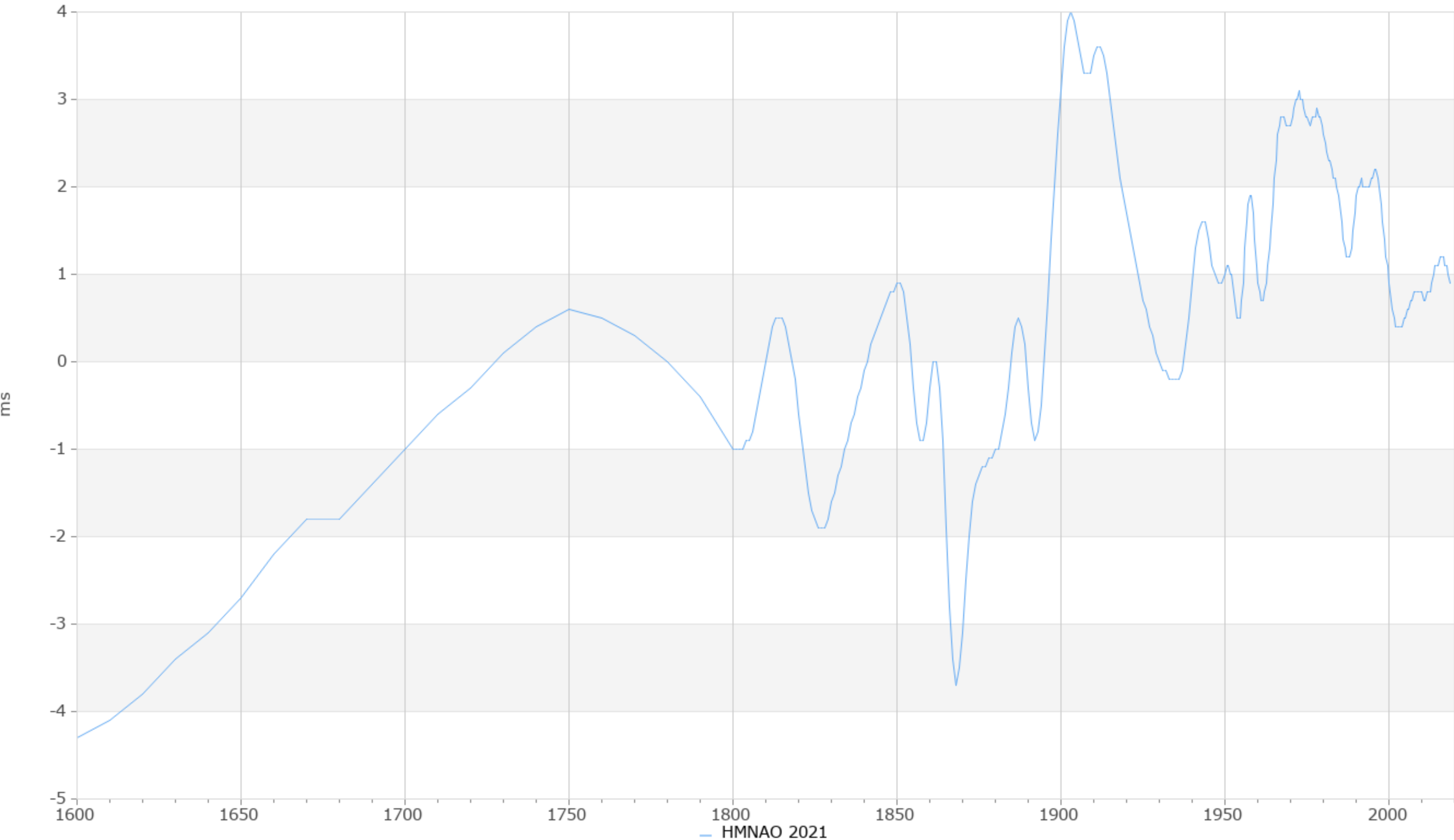
LOD / 86400 s SI
