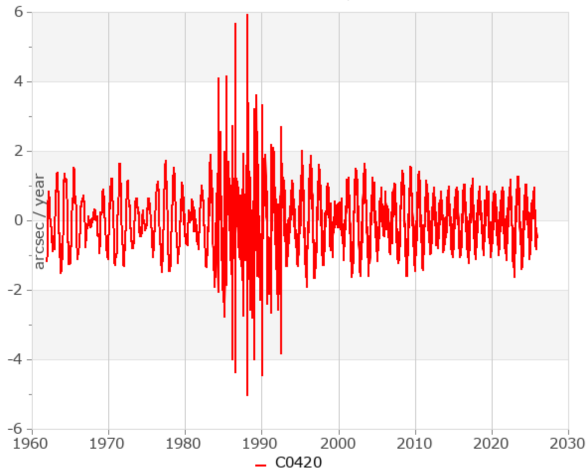
Polar coordinate x/dt
