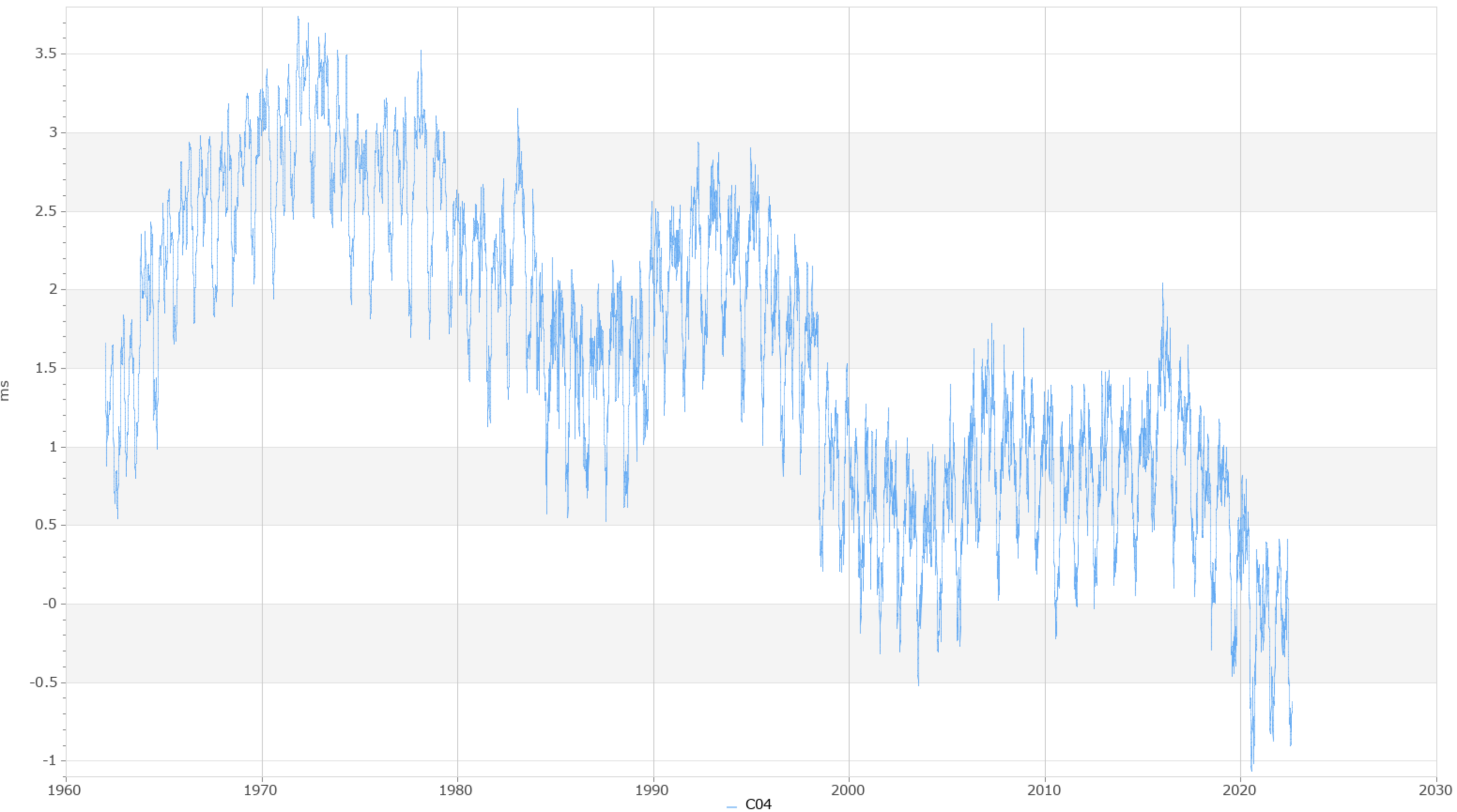
LOD / 86400 s SI
