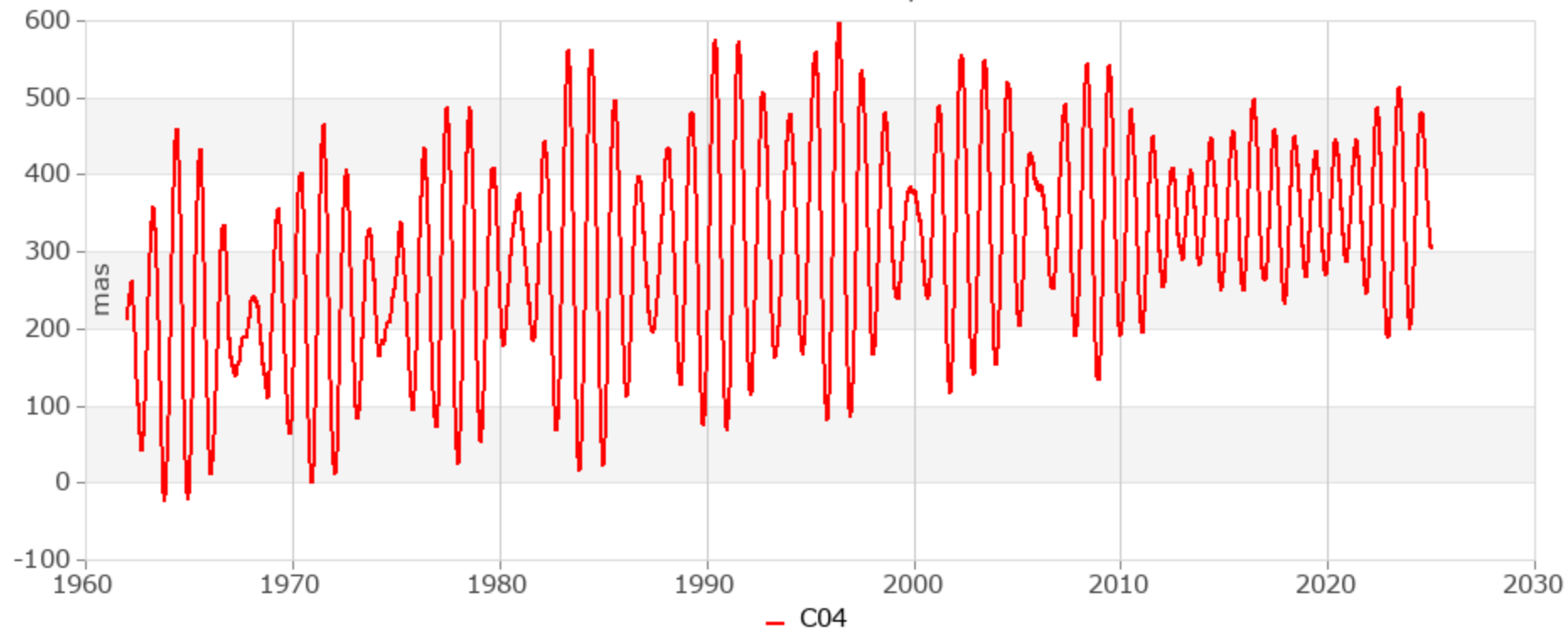
Polar coordinate y
