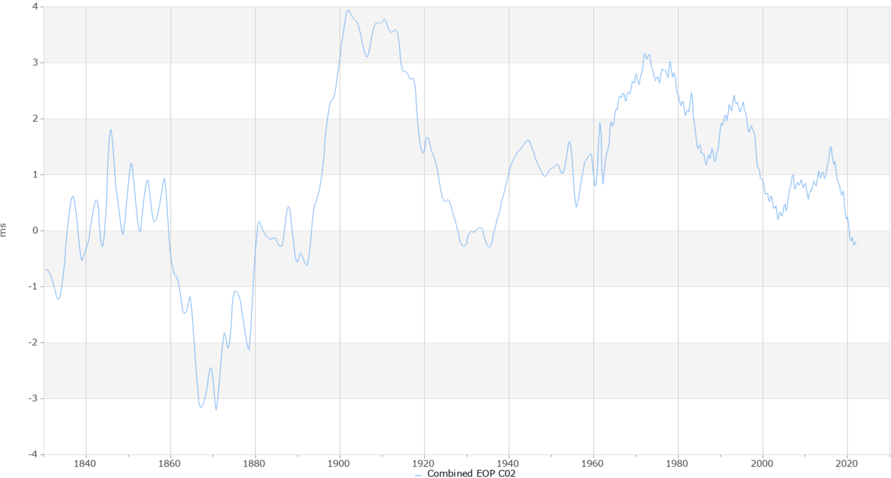
Durée du jour / 86400 s SI
