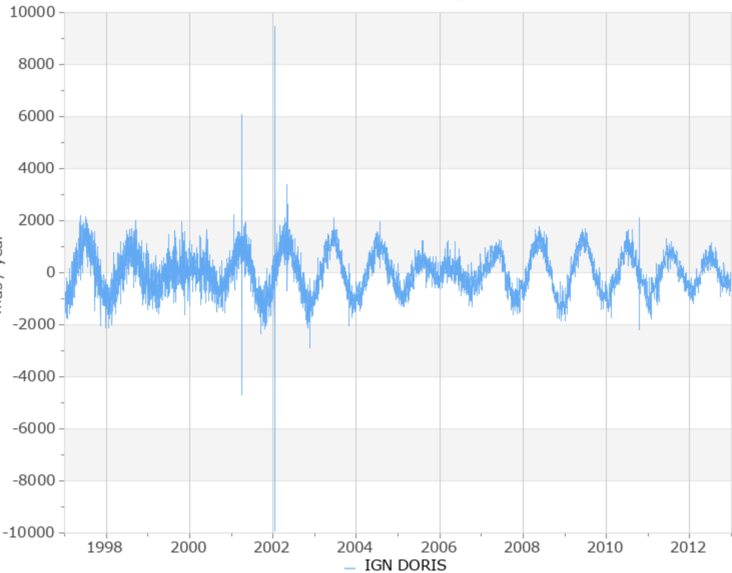
Polar coordinate x /dt
